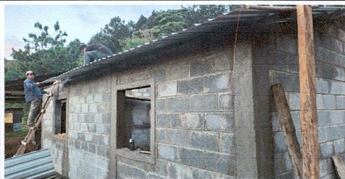
Foto: 6 MEJORAMIENTO MODULO DE AULA TIPO PORTICO, COLOCACIÓN DE LÁMINA TROQUELADA CALIBRE 26
